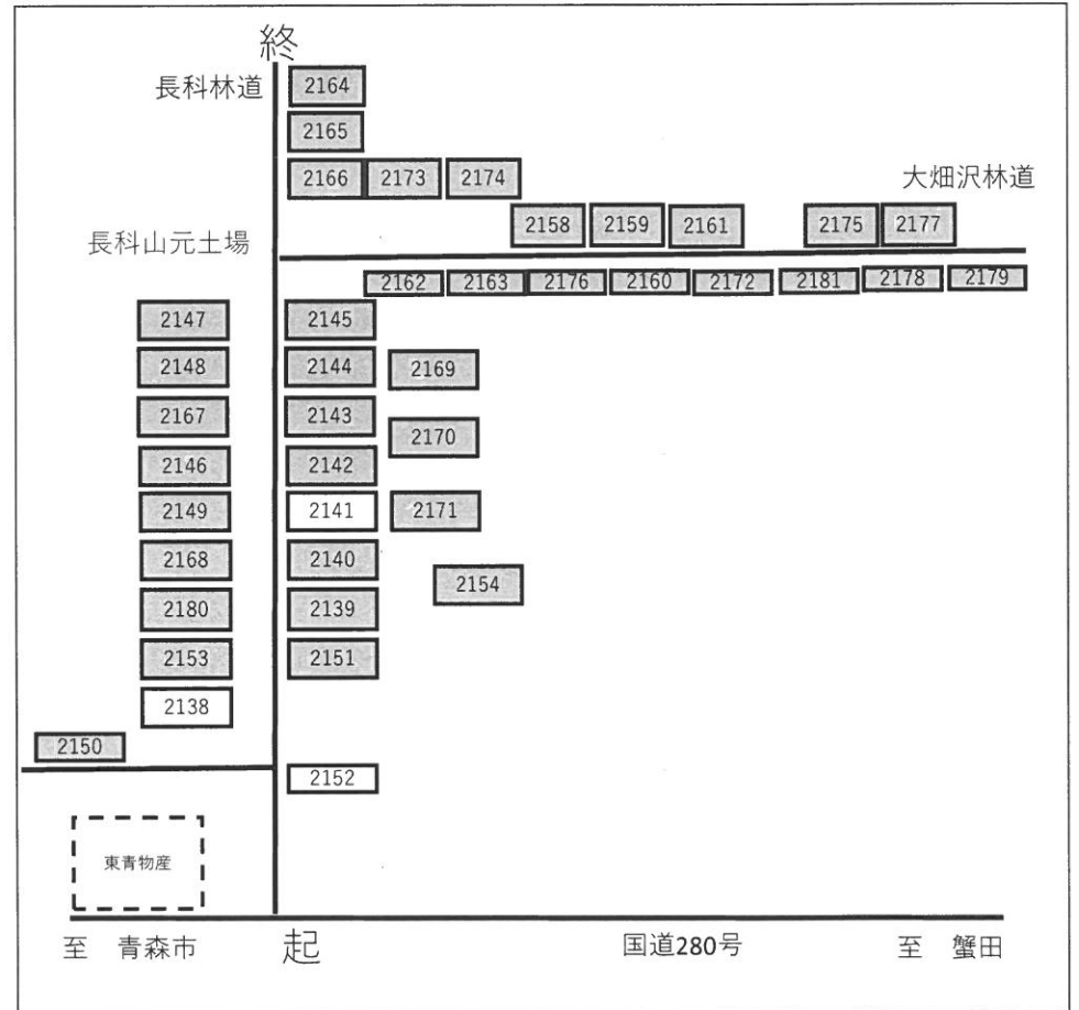
巻立位置図
